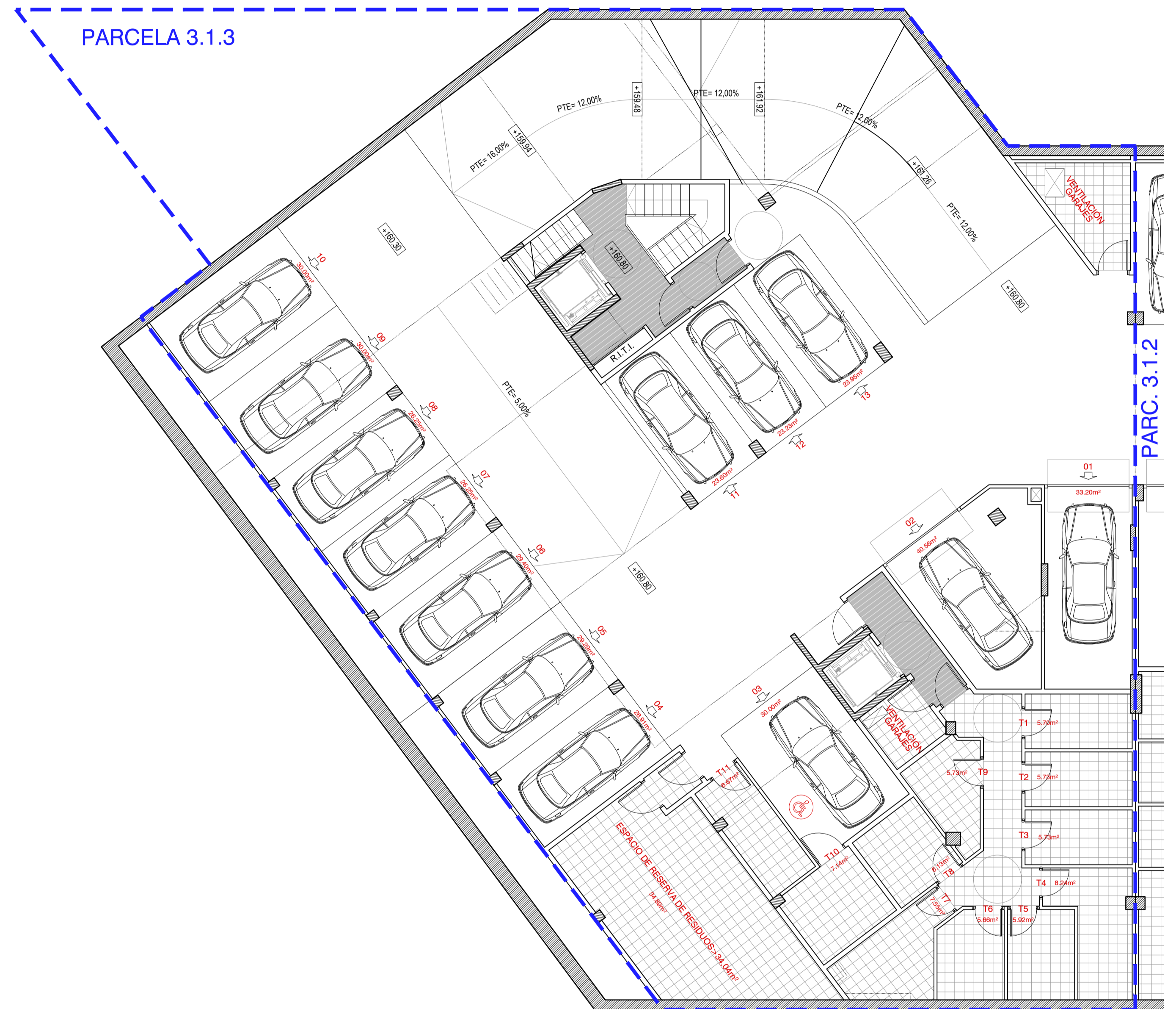
PLANTA SÓTANO -1
