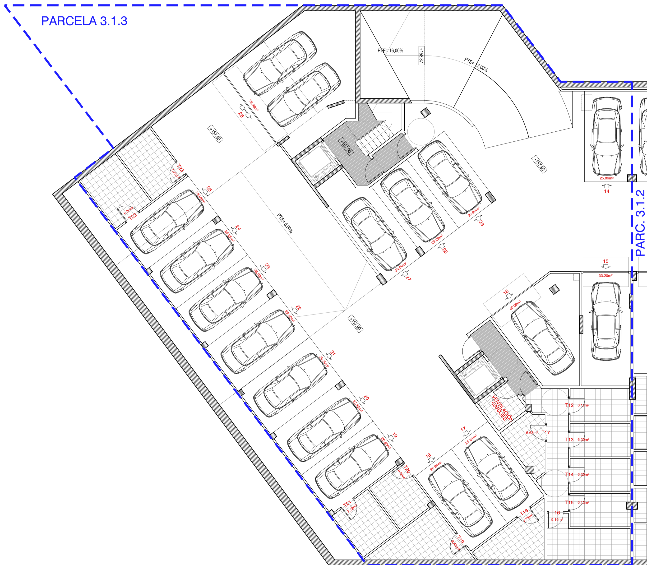
PLANTA SÓTANO -2
