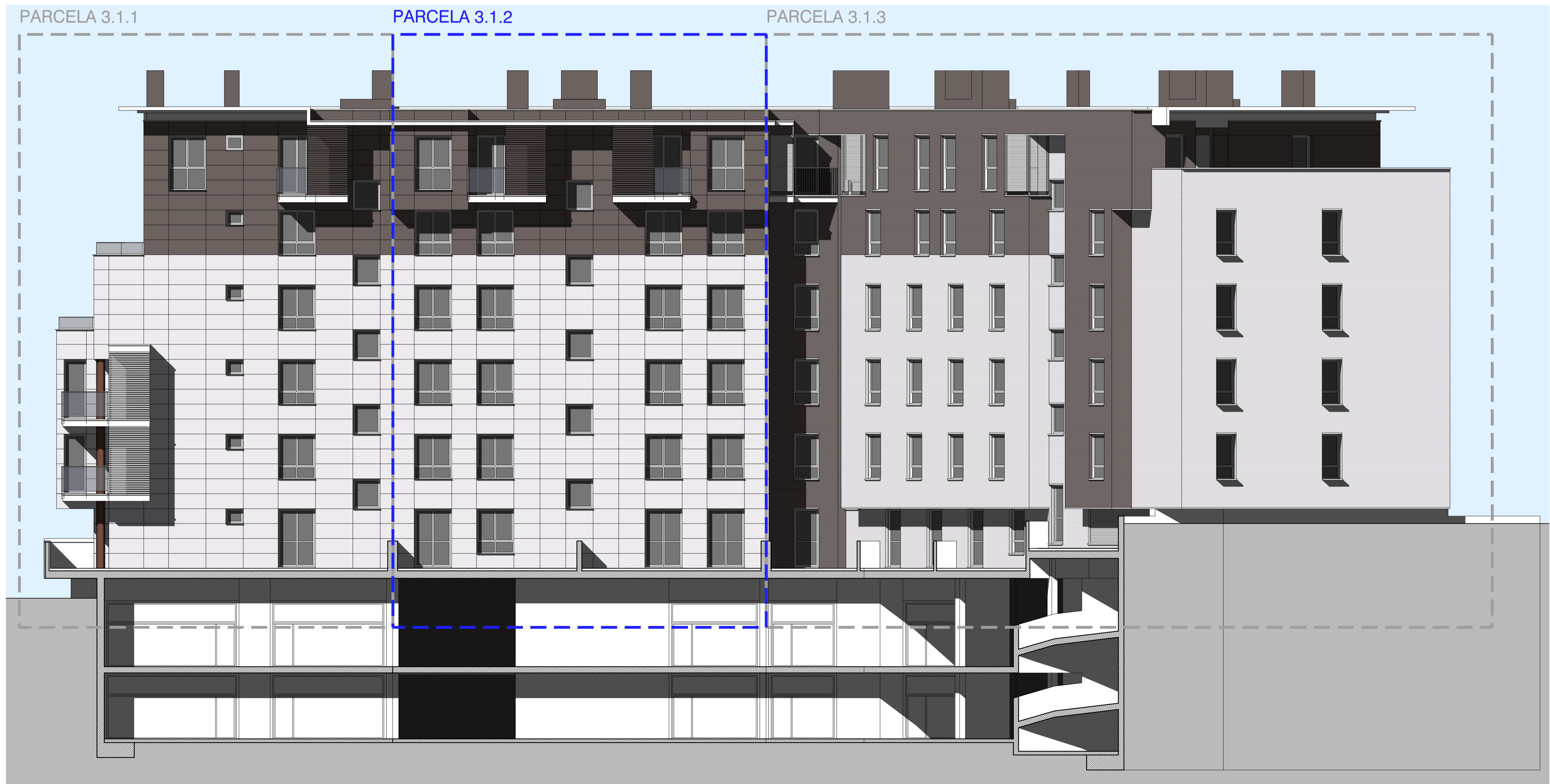
ALZADO NORTE
