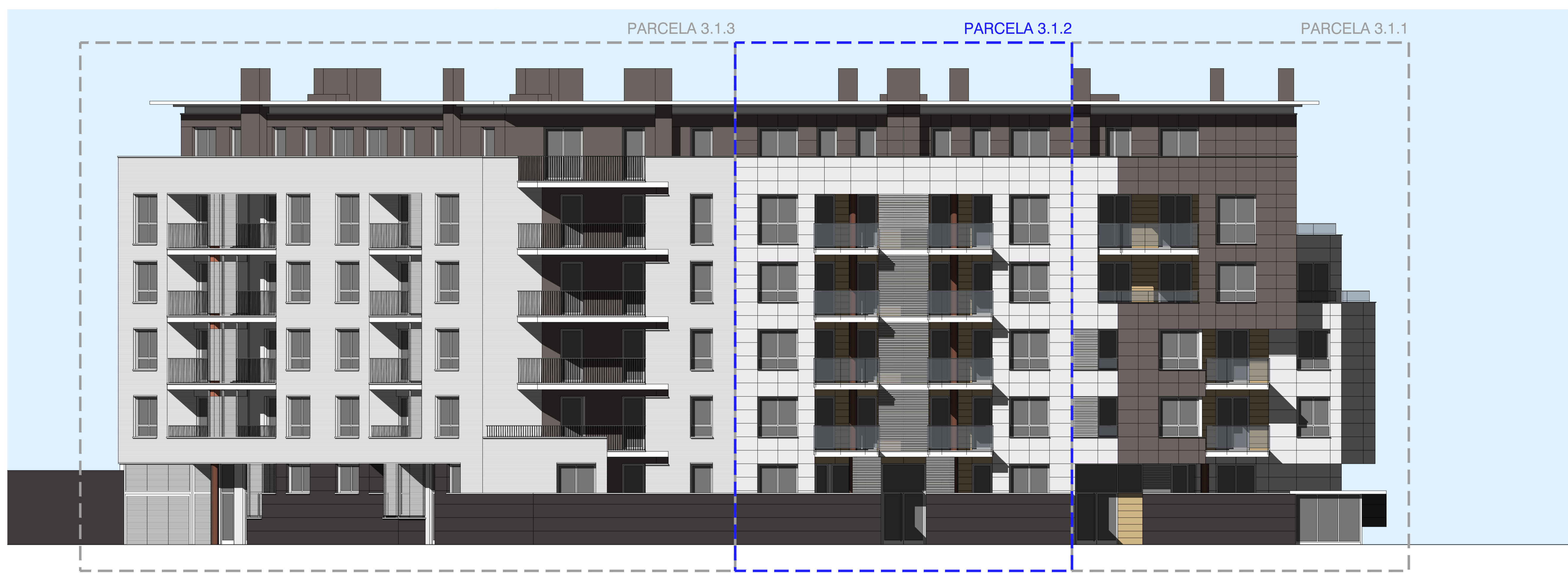
ALZADO SUR
